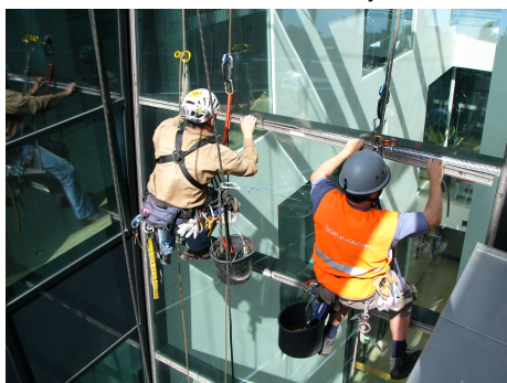
Zasklívání fasád a montáž lišt na budově Arbeiterkammern, Vídeň
